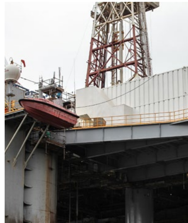
POSICIONAMENTO FINAL DO MÓDULO A 50 M DA LINHA D'ÁGUA
