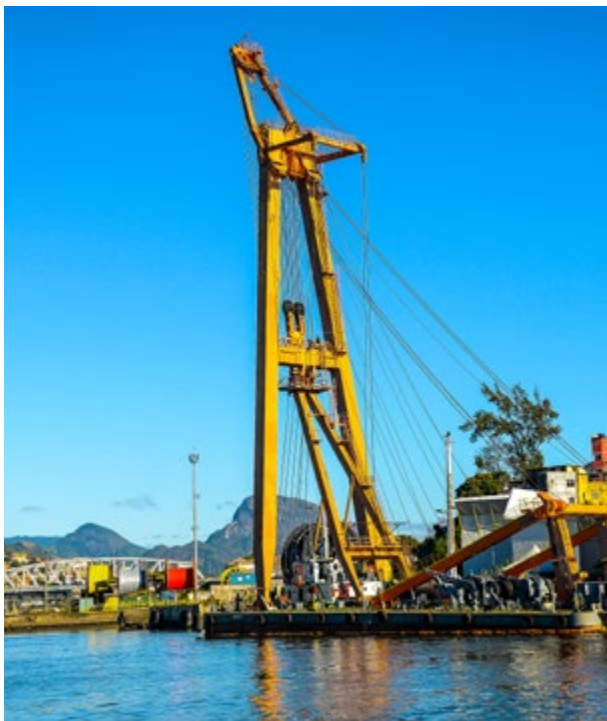
MANUTENÇÃO DA LANÇA DA CÁBREA AMAPÁ - TECHNIP
